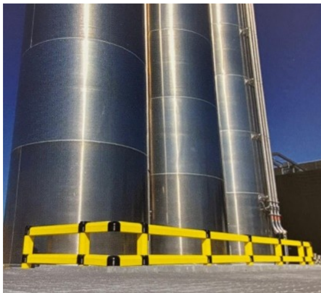
Bijschrift foto: Aanrijdbeveiliging in een opvallende kleur van ca. 1.10 m. hoogte.
